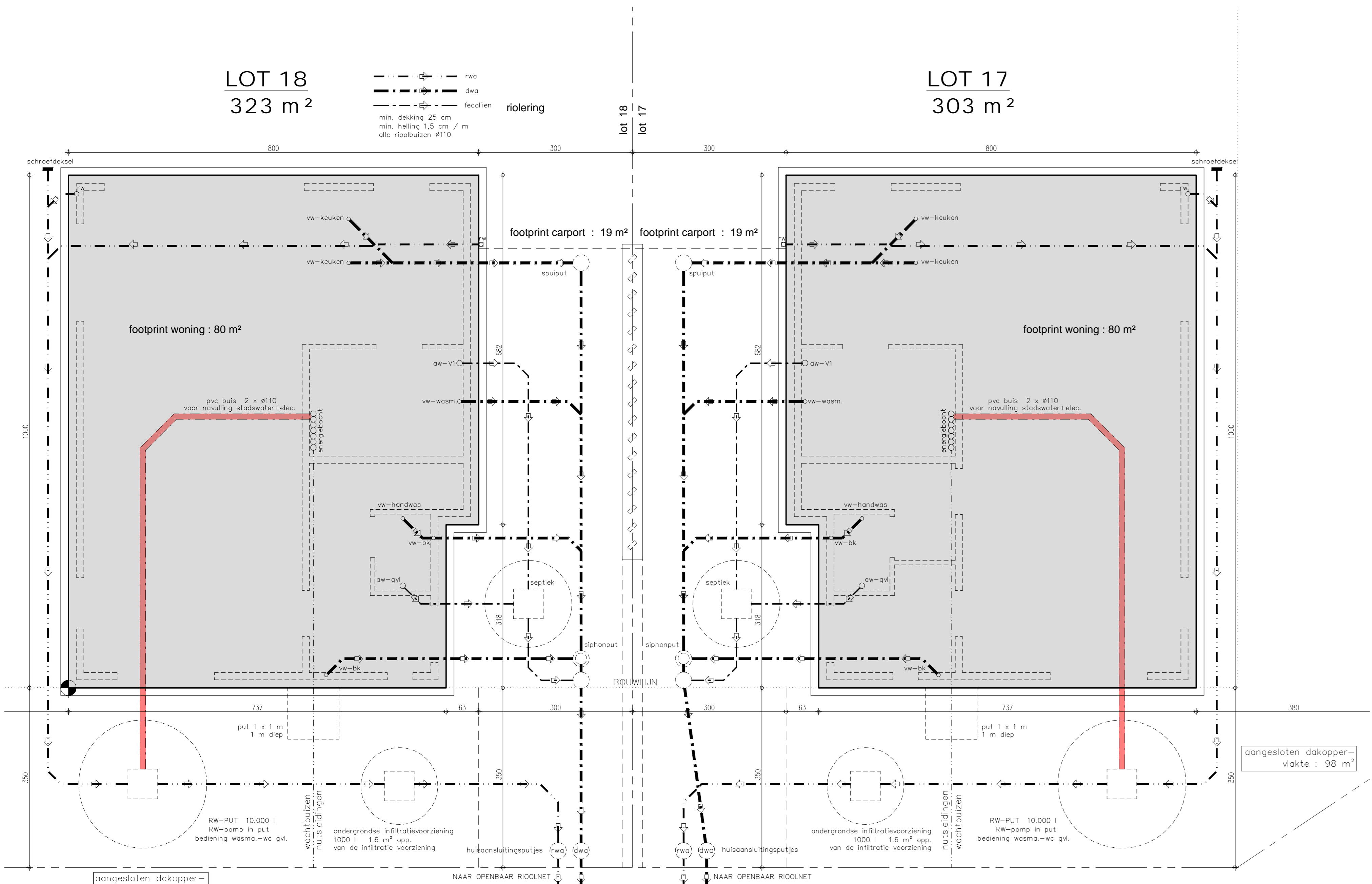
ONDERGROND - RIOLERING 1/50
