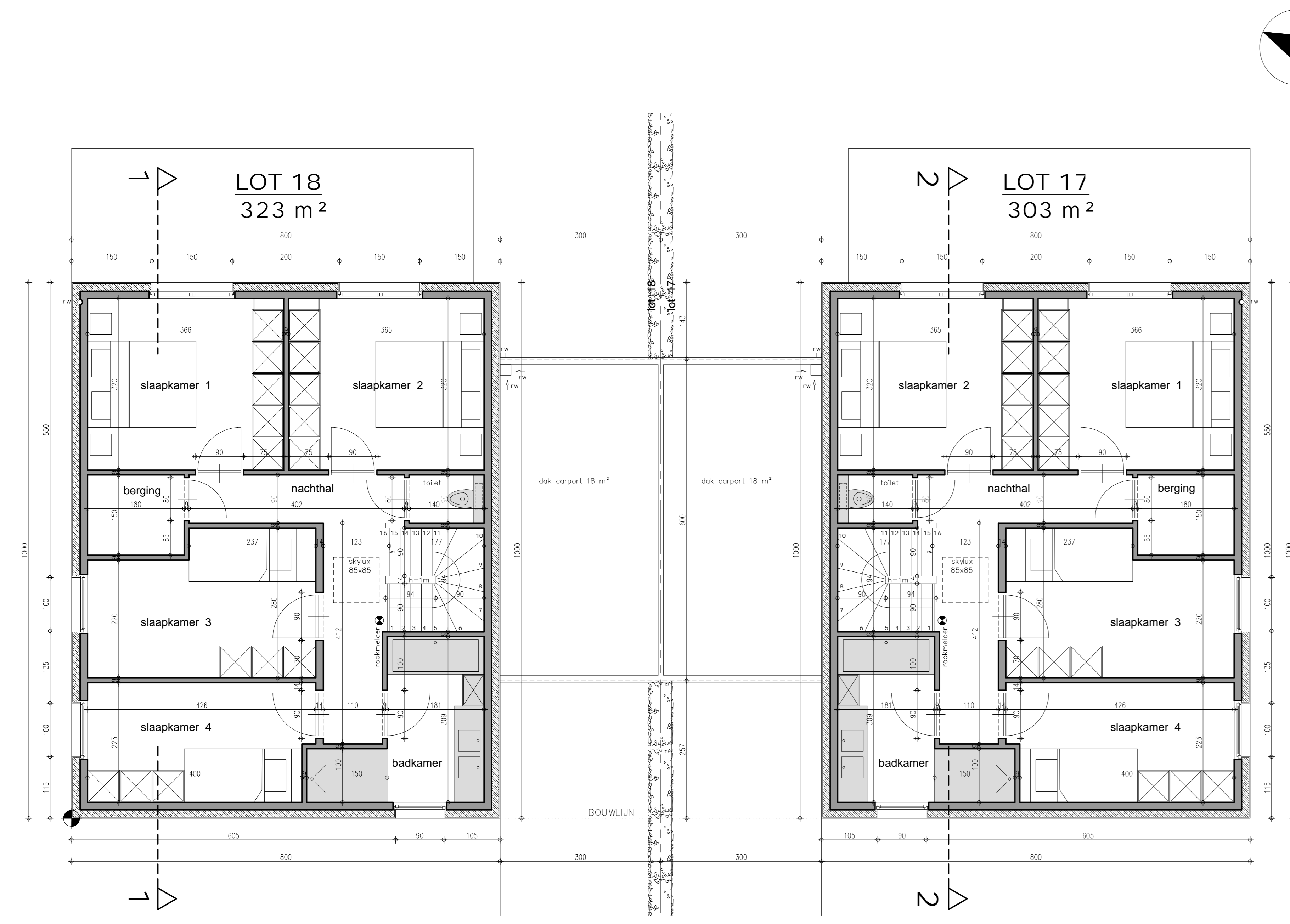
VERDIEPING 1 1/50
