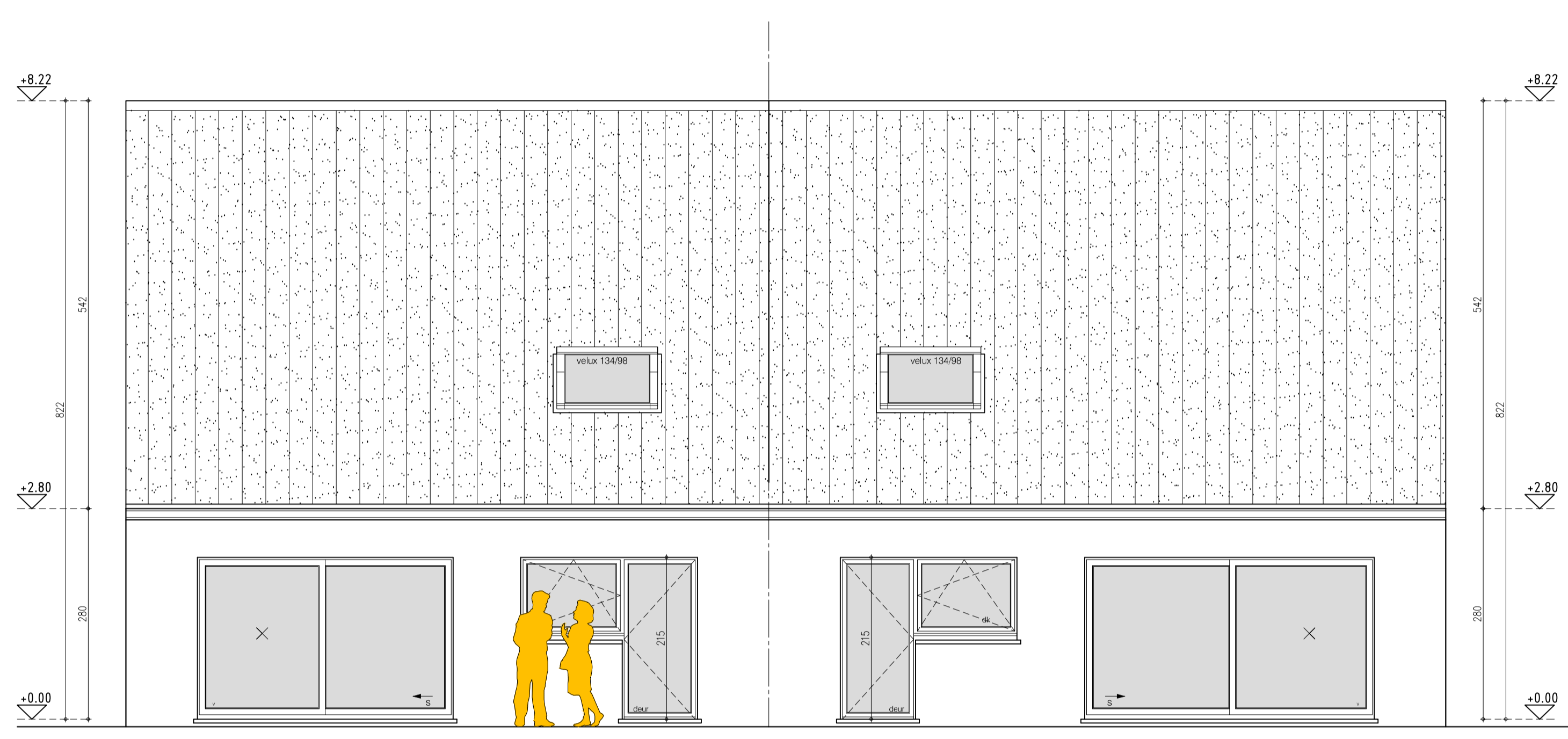
achtergevel lot 29
