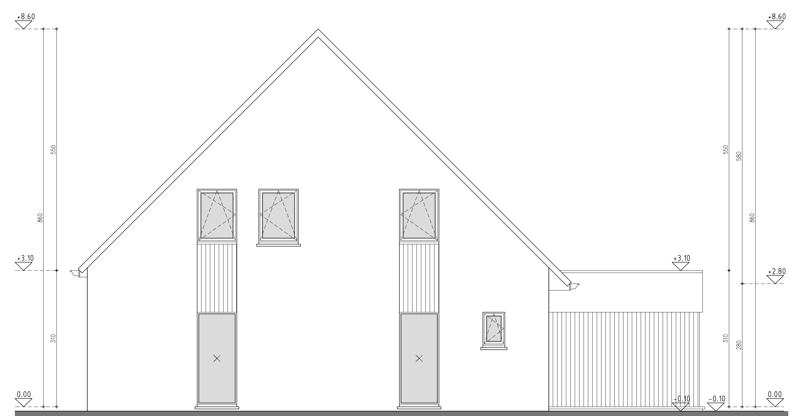
zijgevel lot 3
