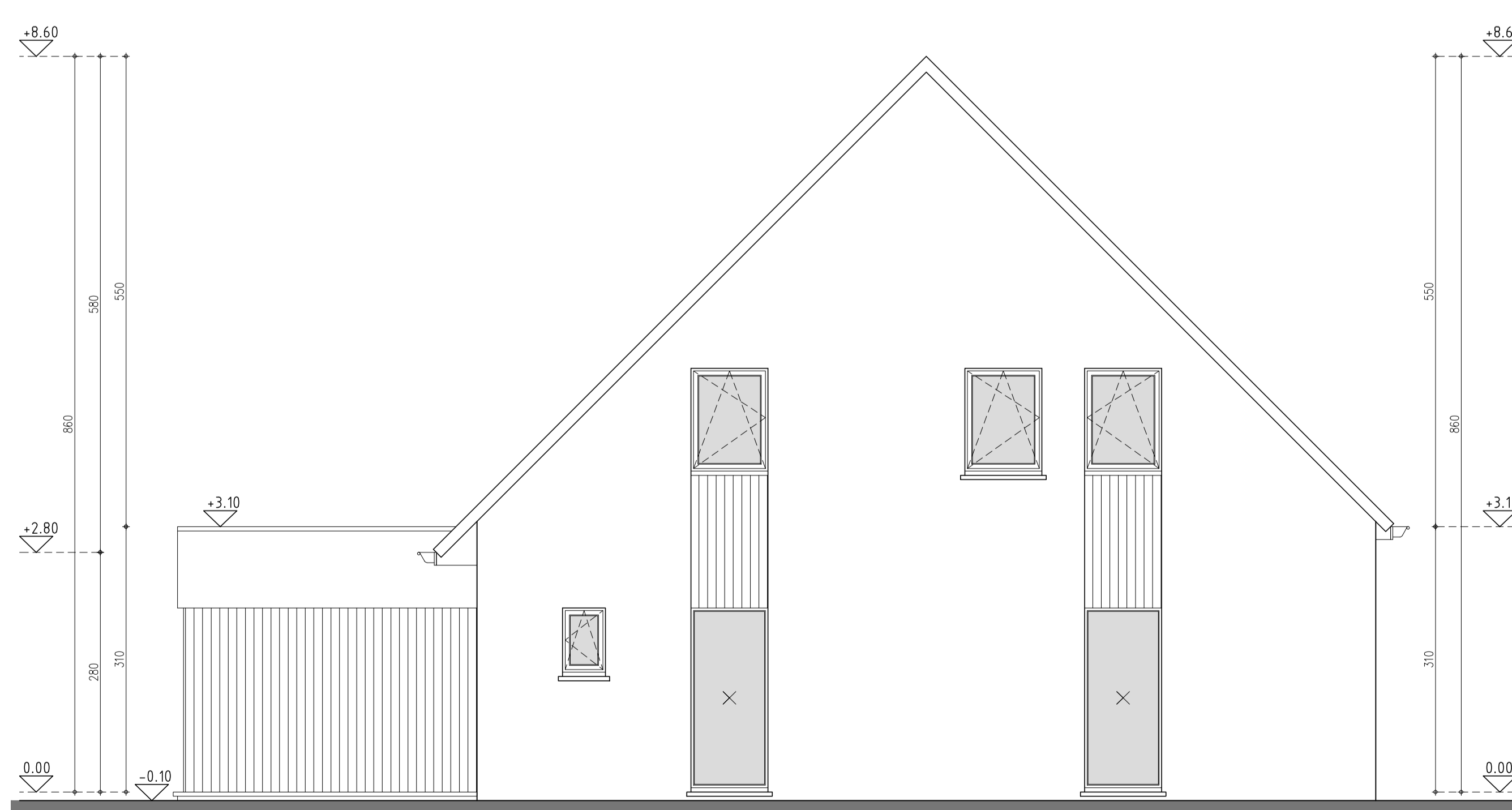
zijgevel lot 4
