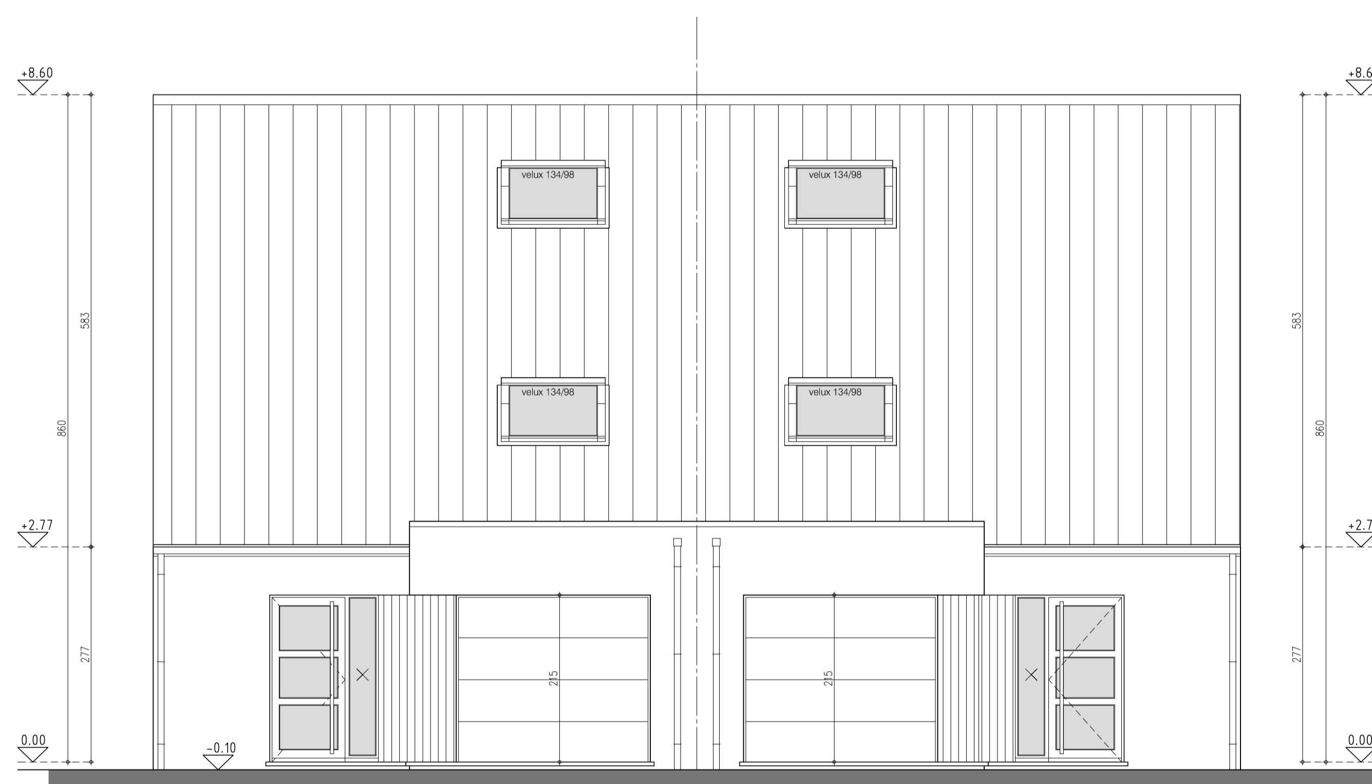
voorgevel lot 3
